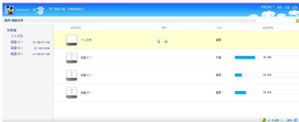
图 5 文件界面
